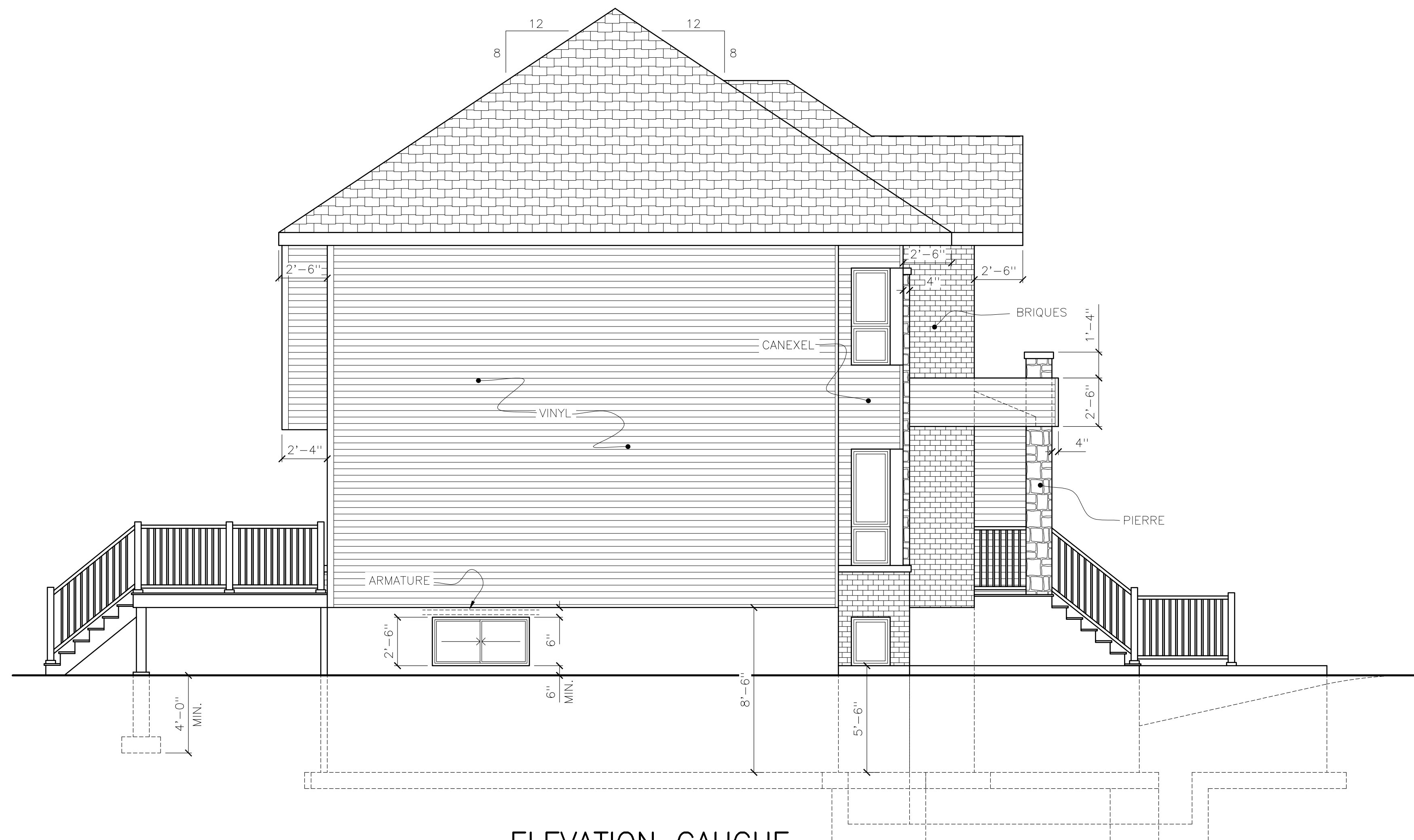
ELEVATION GAUCHE
